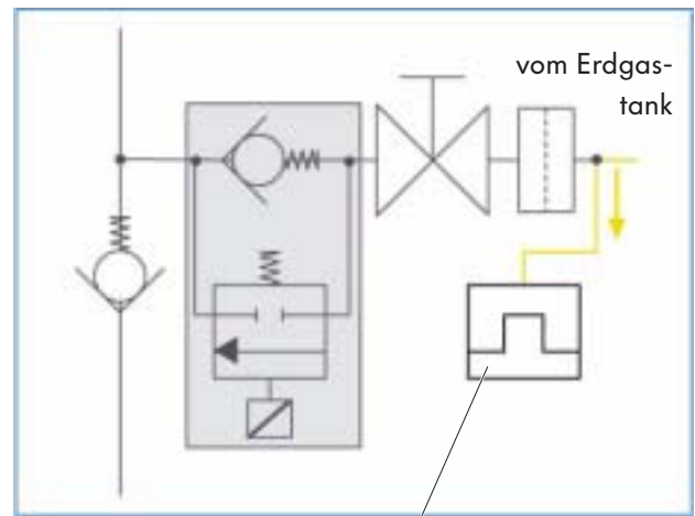
Schmelzlotsicherung
