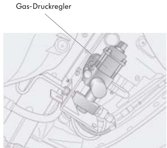
Darstellung ohne Kunststoffabdeckung um den Gas-Druckregler
